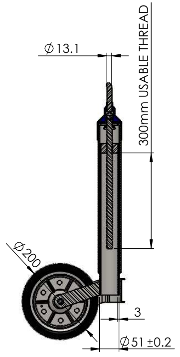
SECTION A-A SCALE 1 : 7
