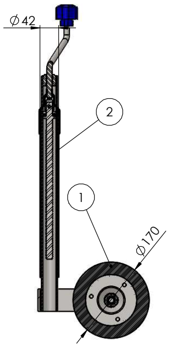
SECTION A-A SCALE 1 : 6
